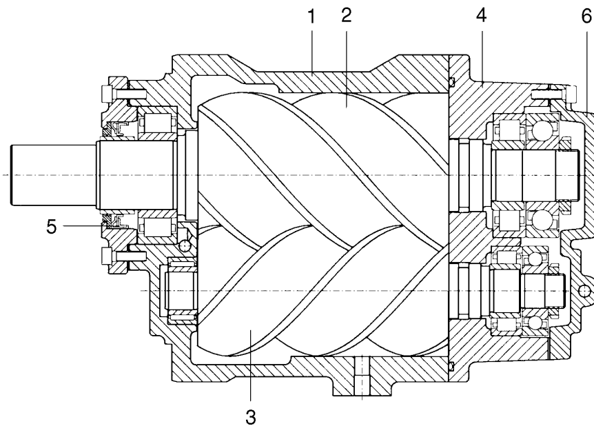
BARE COMPRESSOR
